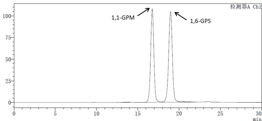
图 1 异麦芽酮糖醇的典型色谱图（1,1-GPM 和 1,6-GPS 的相对保留时间分别约为 1.0 和 1.2。）
