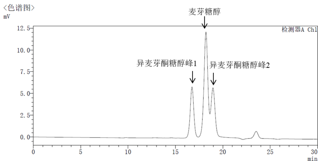
图 2 甘露醇有关物质项下系统适用性溶液 2 的典型色谱图（三个峰分别是异麦芽酮糖醇第一个峰、麦芽糖醇、异麦芽酮糖醇第二个峰。）
