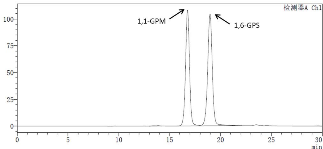
图 1 异麦芽酮糖醇的典型色谱图
